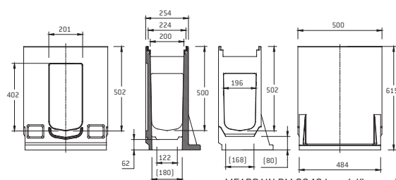
MEADRIN DM 2040 horní díl vpusti
