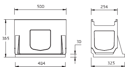
MEADRIN DM 2000 horní díl vpusti
